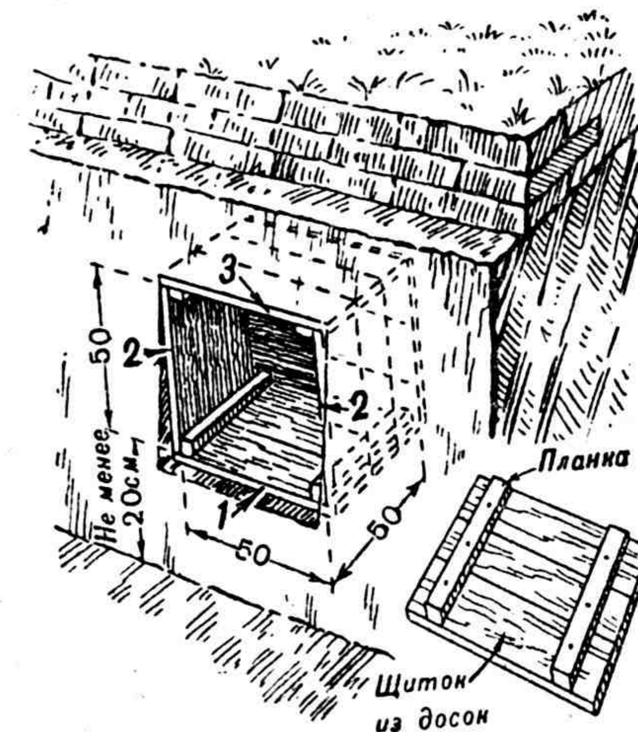
Рис. 13. Ниша для боеприпасов, одетая досками Время на оборудование — 2 часа
