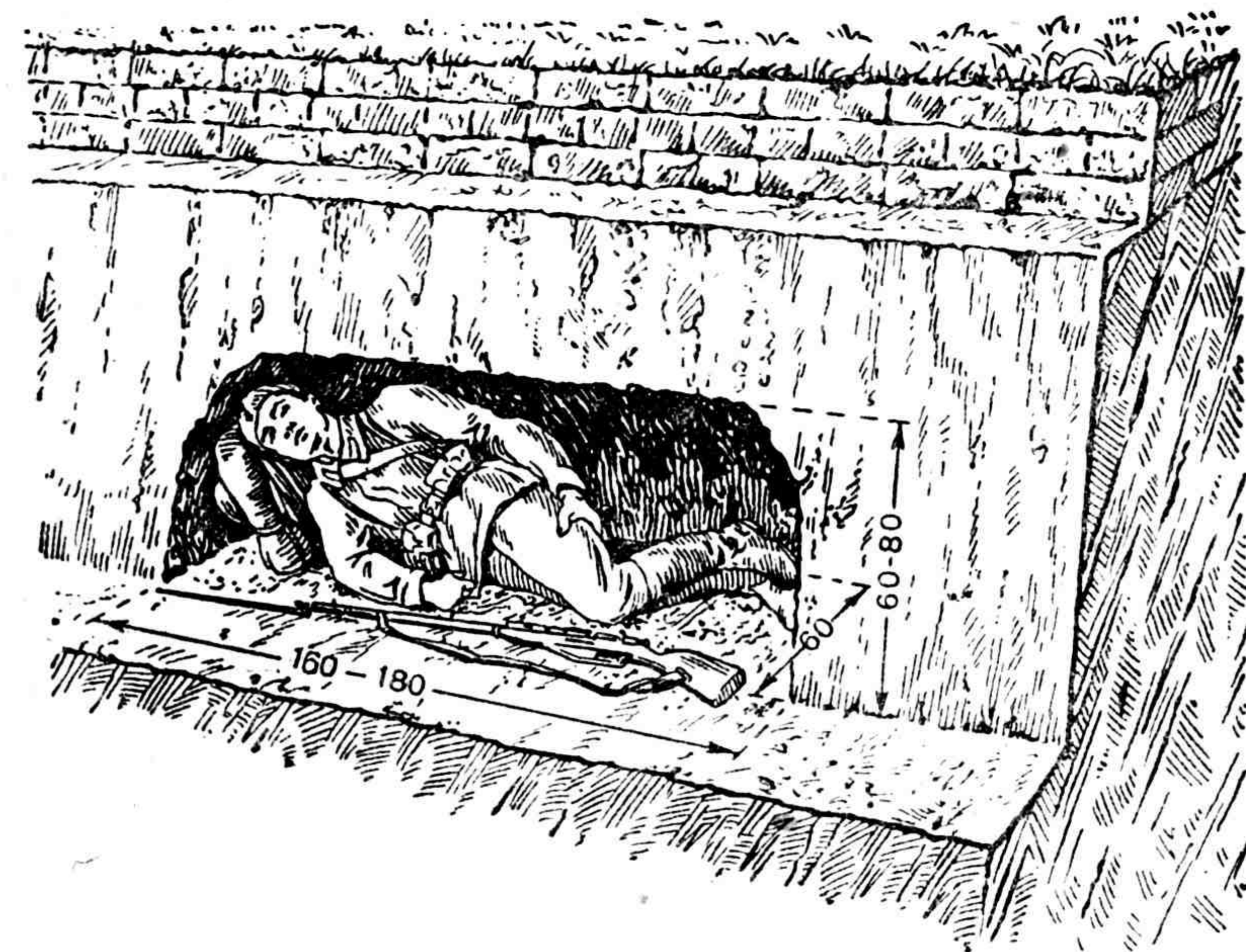
Рис. 15. Ниша для бойца в твердом грунте Время на выделку — 4 часа
