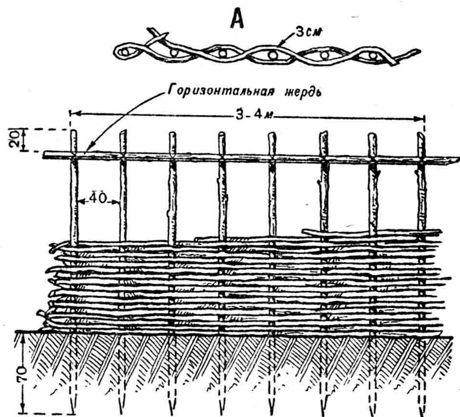
Рис. 28. Изготовление плетня: А — плетение в одну ветвь
