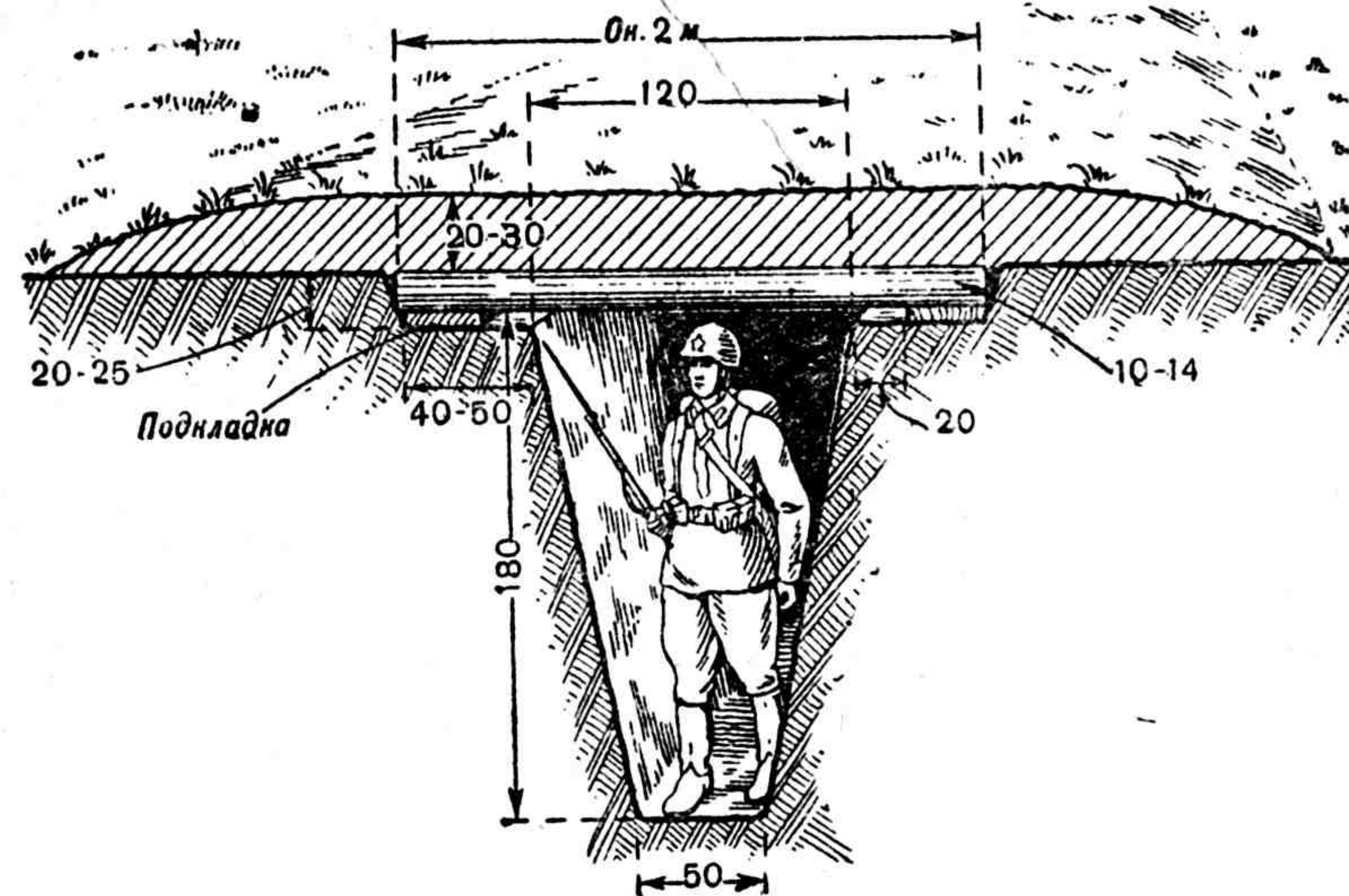
Рис. 22. Устройство перекрытия над ходом сообщения Время на устройство 1 пог. м одним бойцом — 1 час
