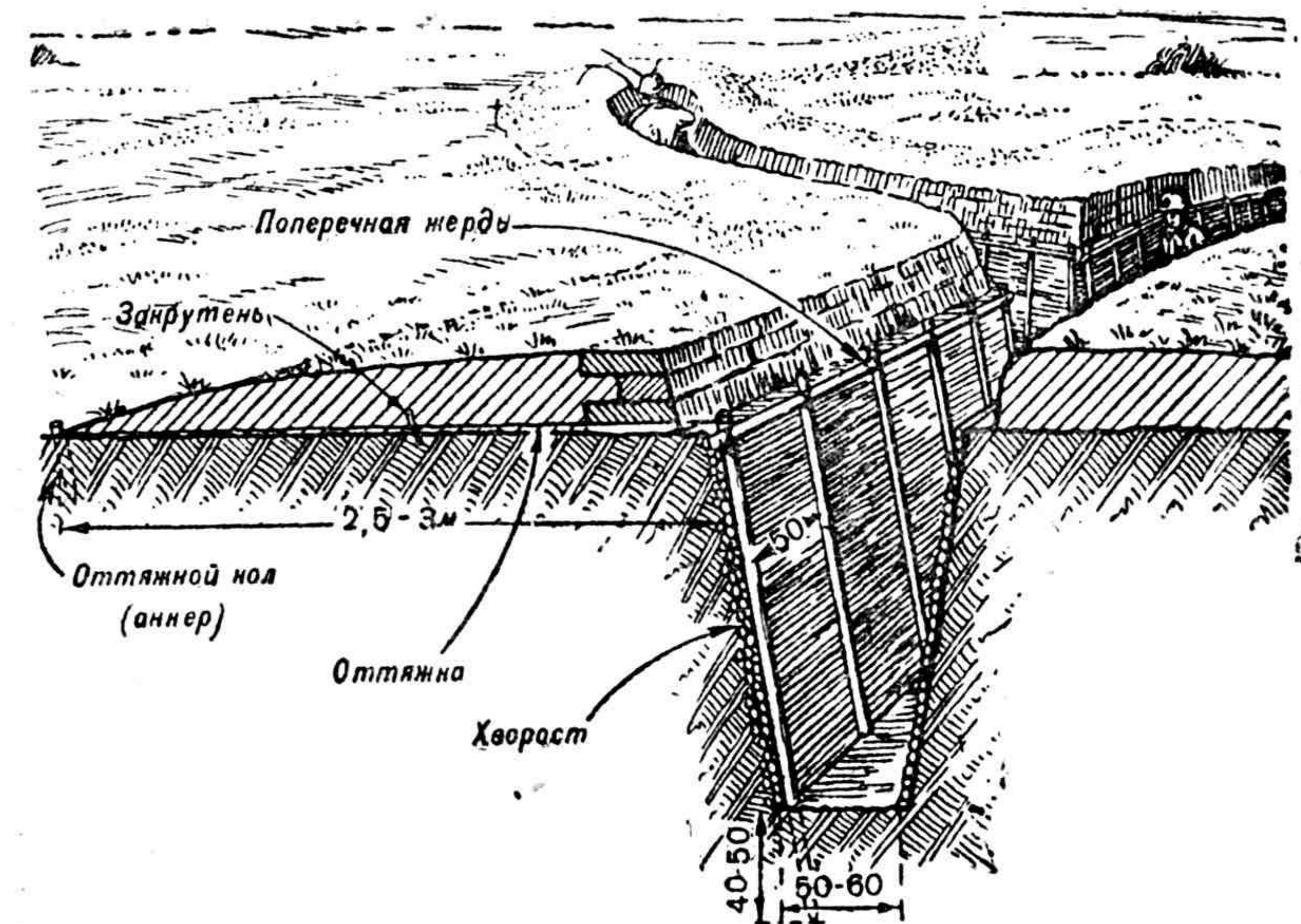
Рис. 27. Окоп, одетый хворостом Два бойца оденут 1 пог. м крутости за 1 час 30 минут
