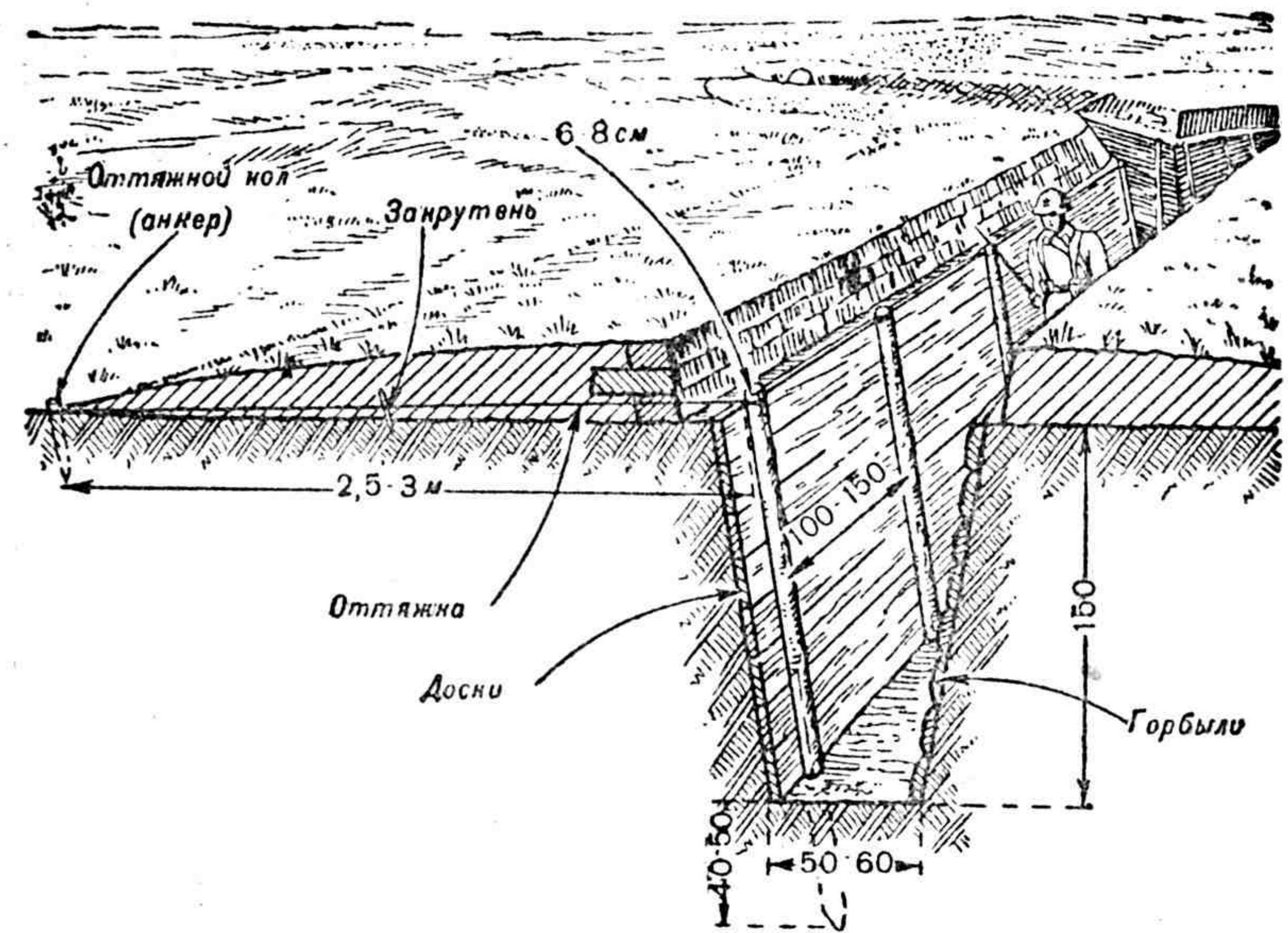
Рис. 26. Окоп, одетый досками Два бойца оденут 1 пог. м крутости за 1 час
