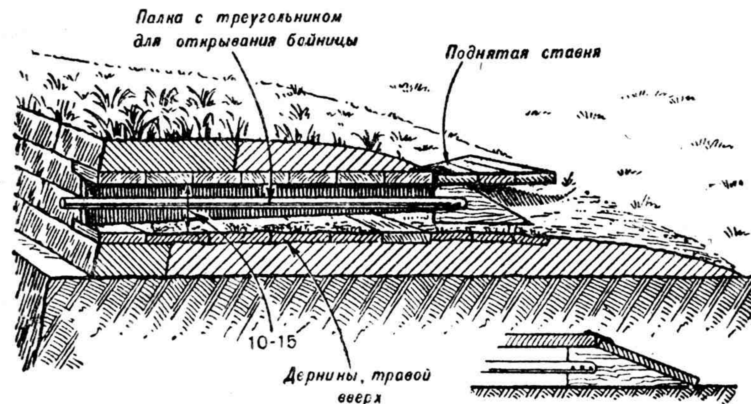
Рис. 11. Устройство поднимающейся ставни бойницы
