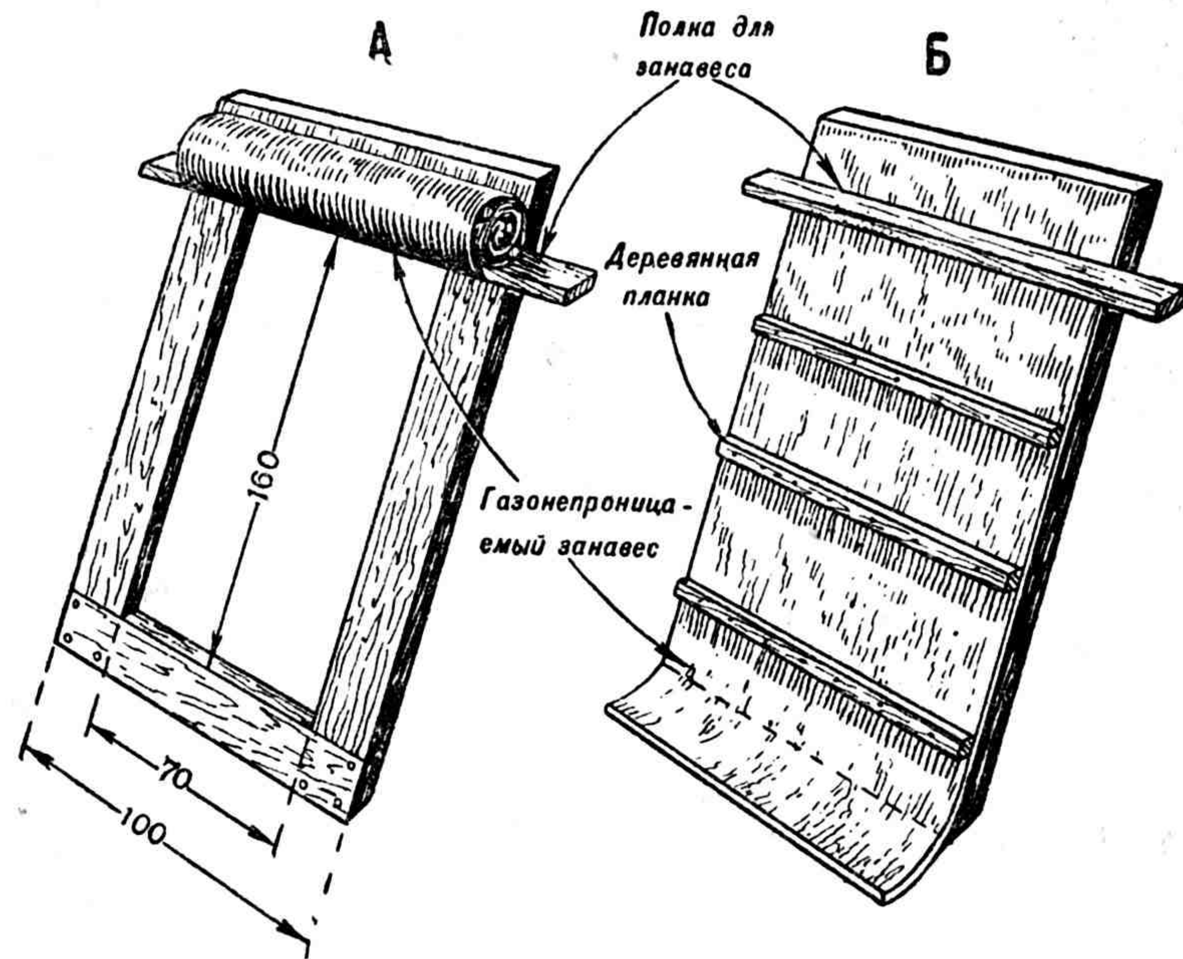
Рис. 41. Устройство газонепроницаемого занавеса: А — занавес открыт; В — занавес закрыт
