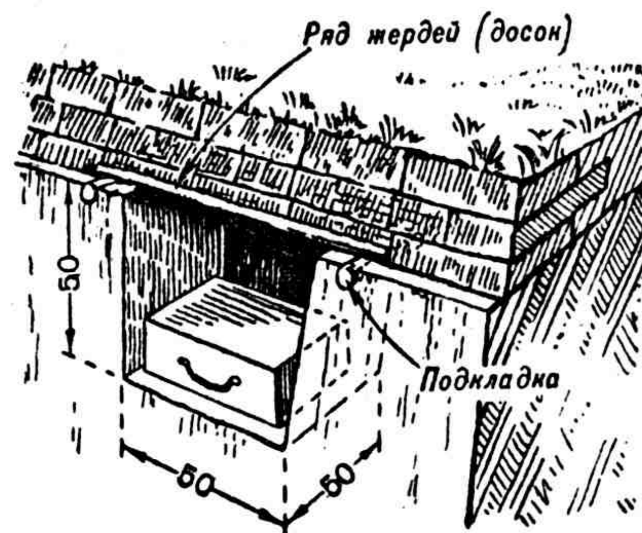
Рис. 12. Ниша для боеприпасов с покрытием из жердей Время на оборудование — 1 час 30 минут
