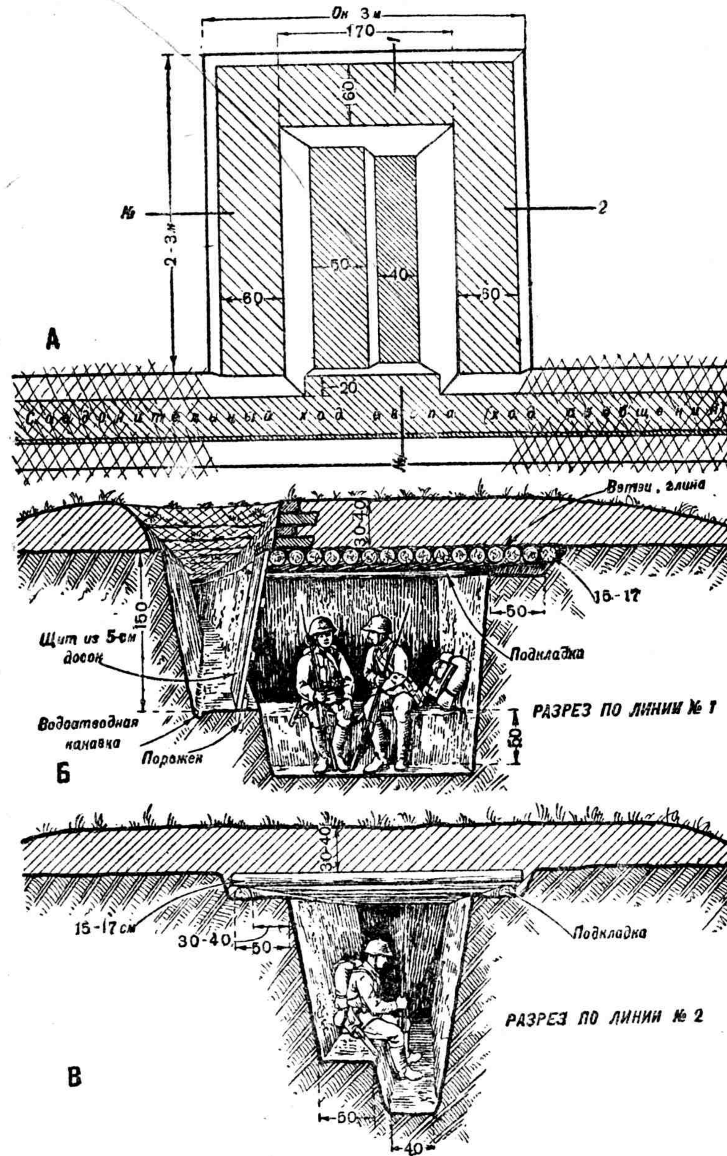
Рис. 24. Подбрустверный блиндаж:
