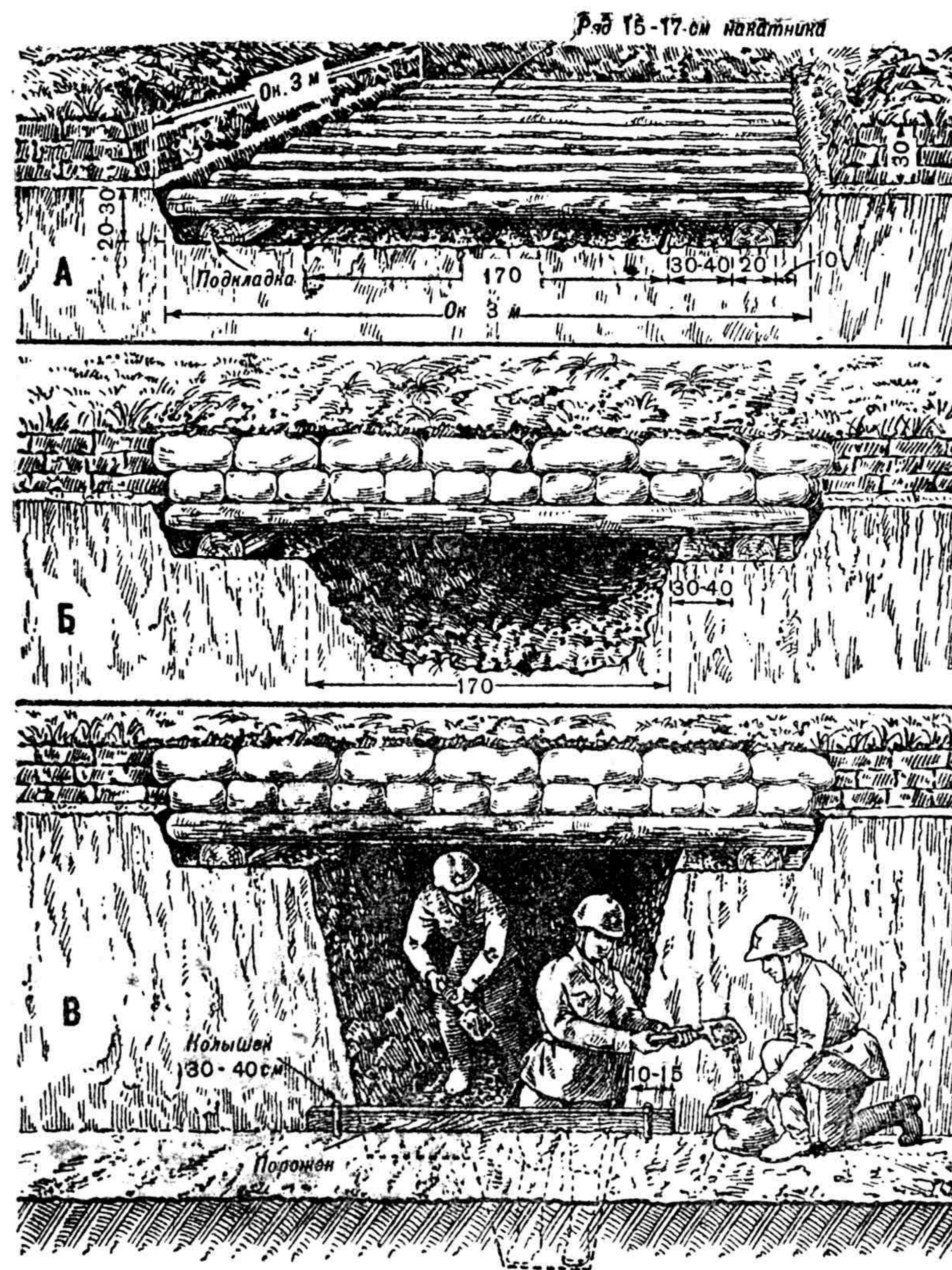
Рис. 25. Отрывка подбрустверного блиндажа в готовом окопе (последовательность работы):
