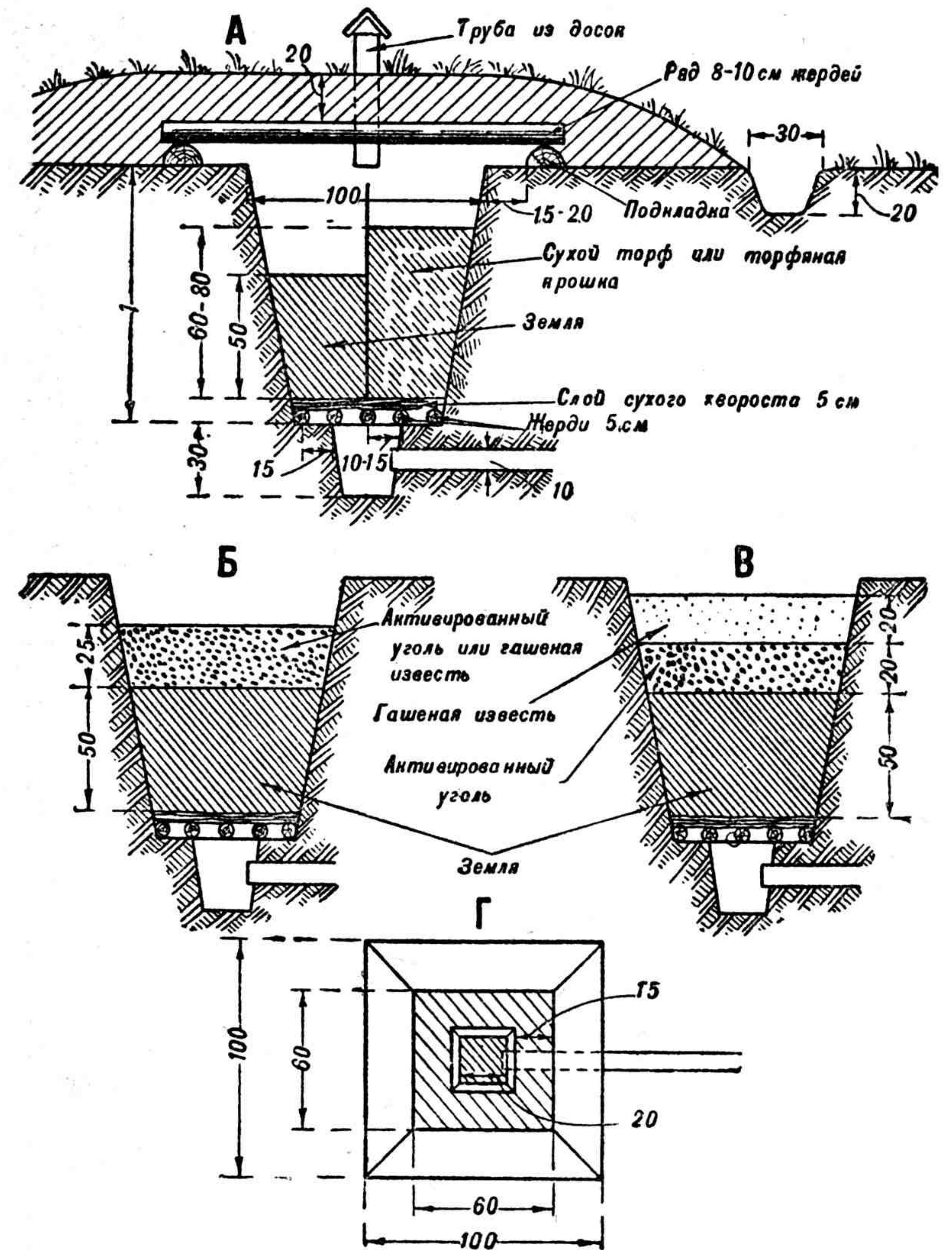
Рис. 42. Устройство фильтра из подручных материалов: А — разрез фильтра из земли или торфа; В и С — разрез фильтра из земли, угля и извести; Г — план фильтра
