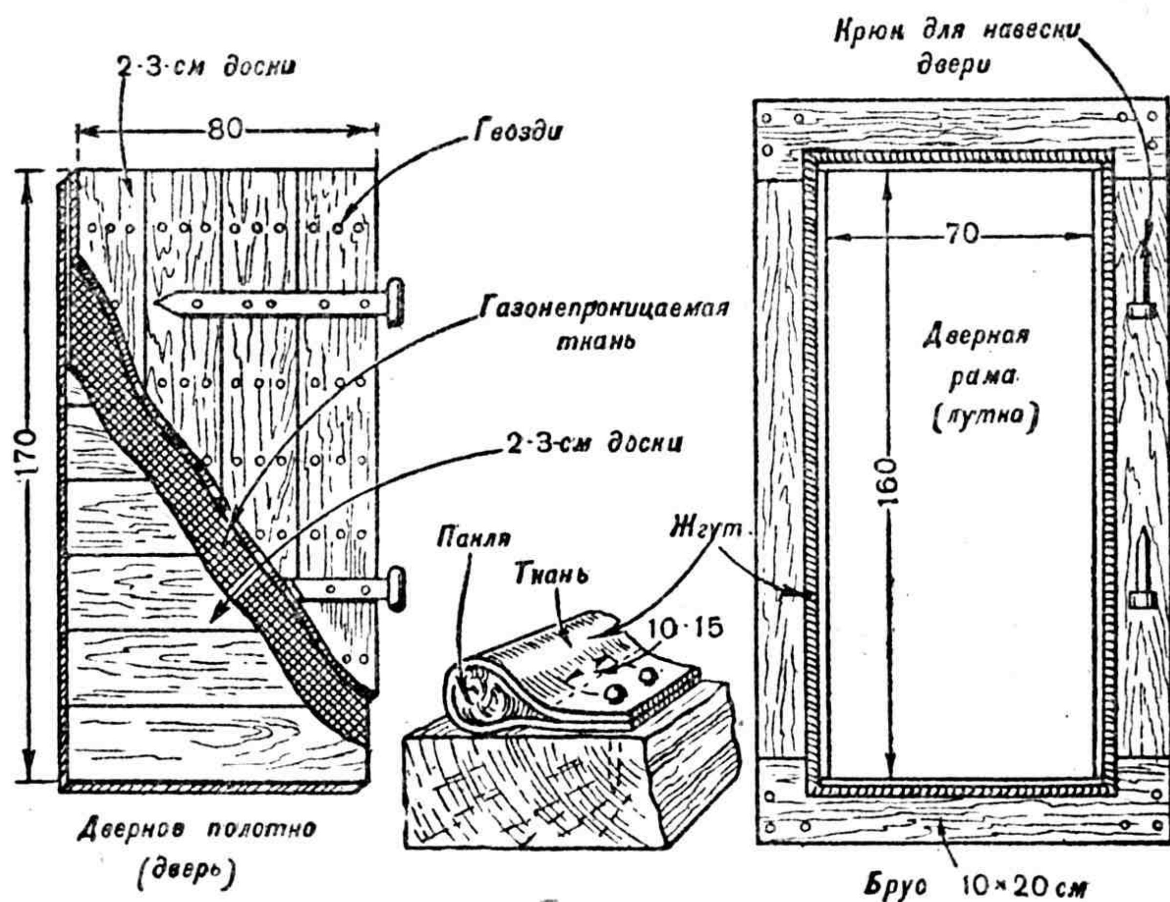
Рис. 39. Устройство герметической (газонепроницаемой) двери
