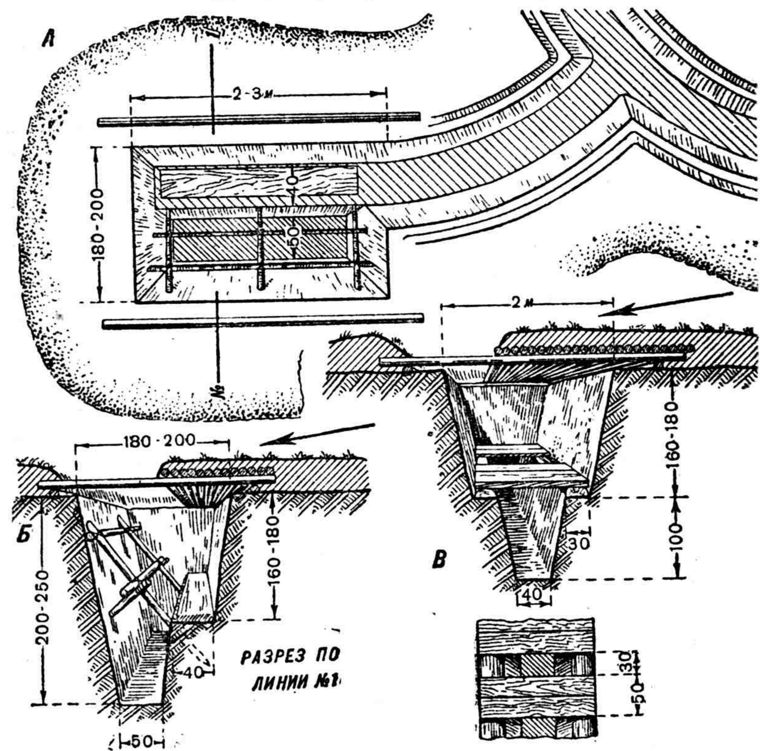
Рис. 34. Устройство отхожего места:
