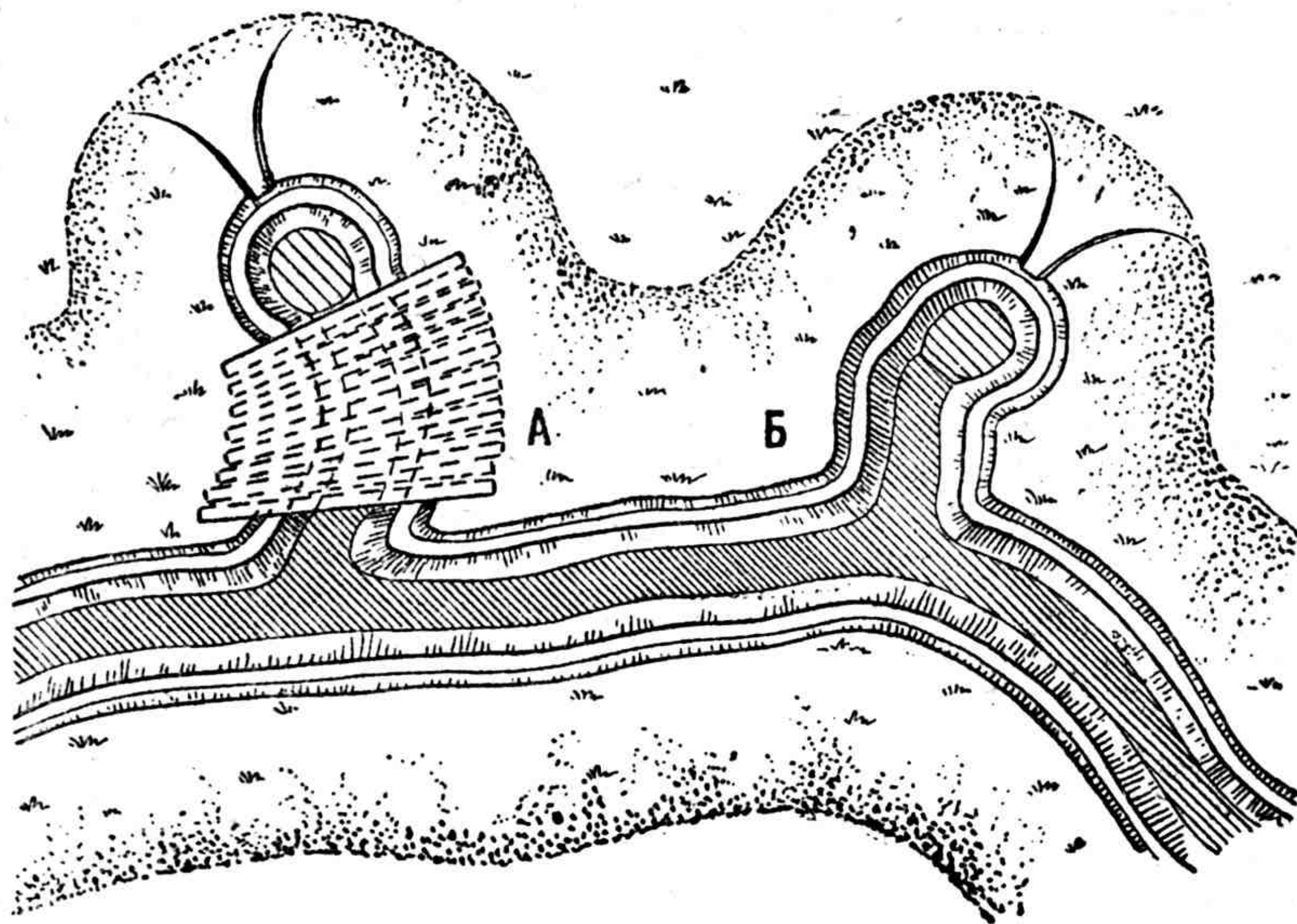
Рис. 21. Перекрытие над окопом: А — перекрытая ячейковая щель; В — неперекрытая ячейковая щель
