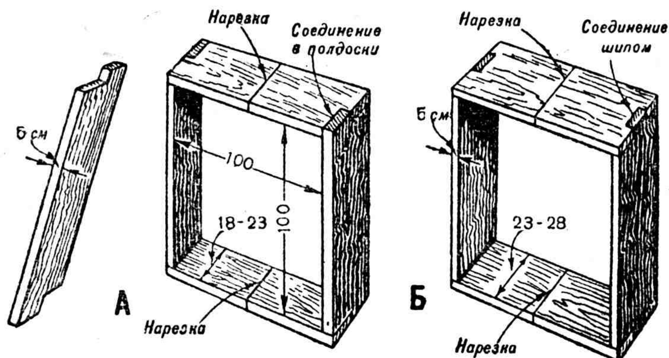
Рис. 16. Готовые рамы из досок для укрепления ниши: А — соединение в полдоски; Б — соединение шипом
