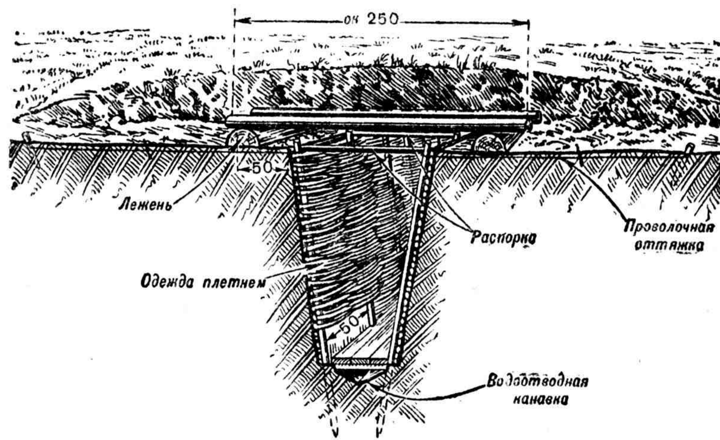
Рис. 36. Поперечный разрез покрытой щели Два бойца за 2 часа 30 минут откоп и перекроют 1 пог. м щели
