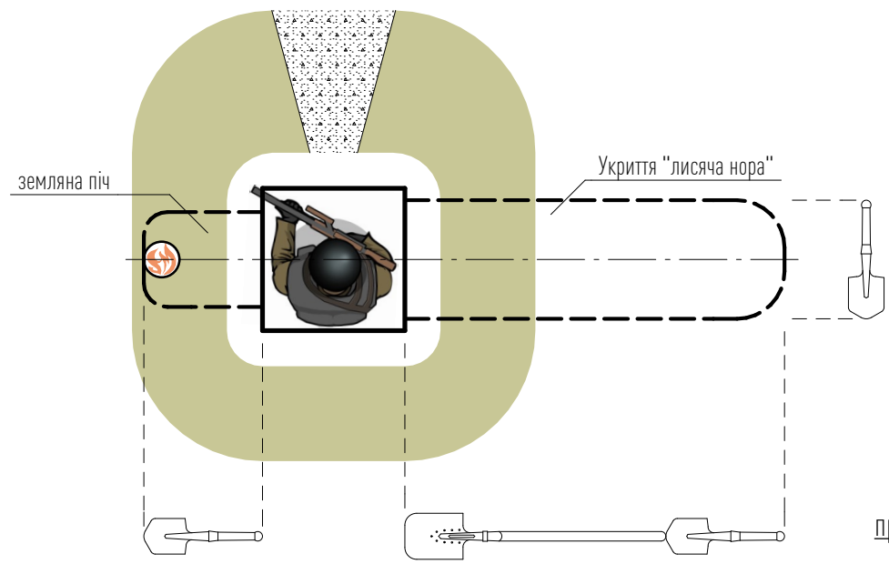
Одиночний квадратний окоп
