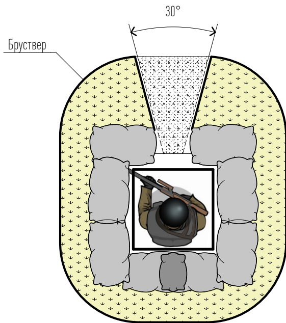
Одиночний квадратний окоп
