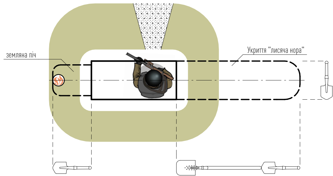
Одиночний прямокутний окоп
