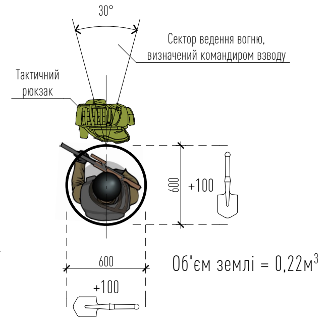
Одиночний окоп "Стакан"
