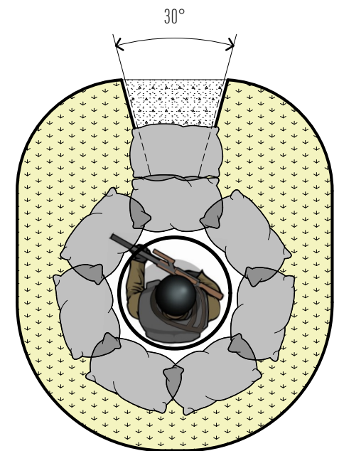
Одиночний окоп "стакан"
