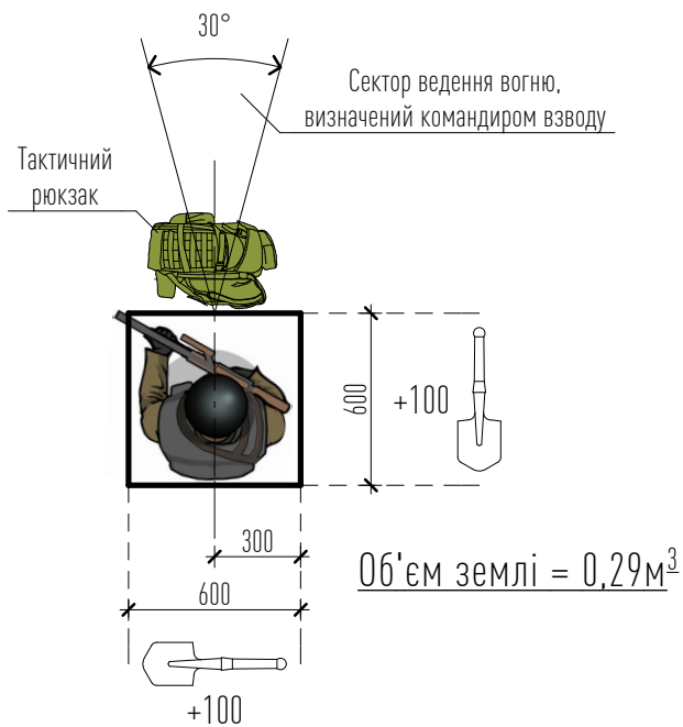
Одиночний квадратний окоп
