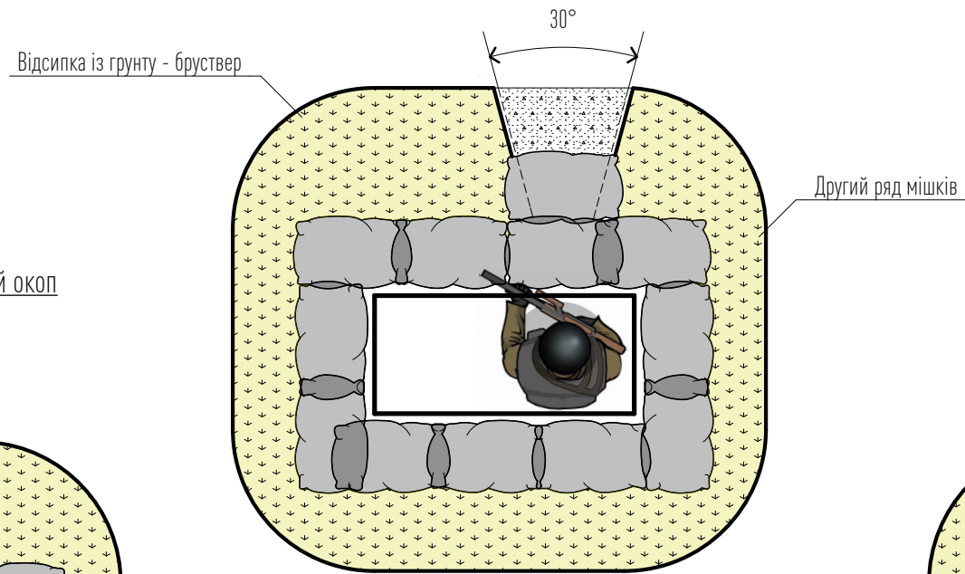
Одиночний прямокутний окоп
