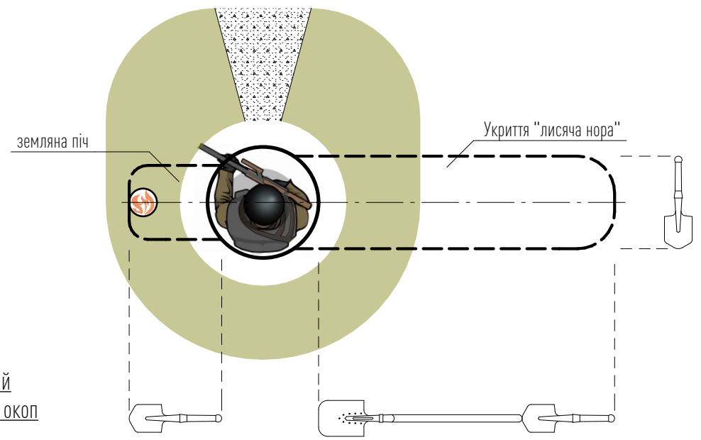
Одиночний окоп "Стакан"
