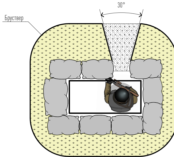
Одиночний прямокутний окоп
